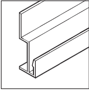
8212 EXTRUSION
